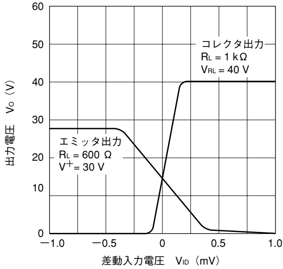
V_O-V_{ID} 特性
