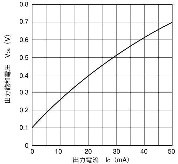
V_{OL}-I_O 特性
