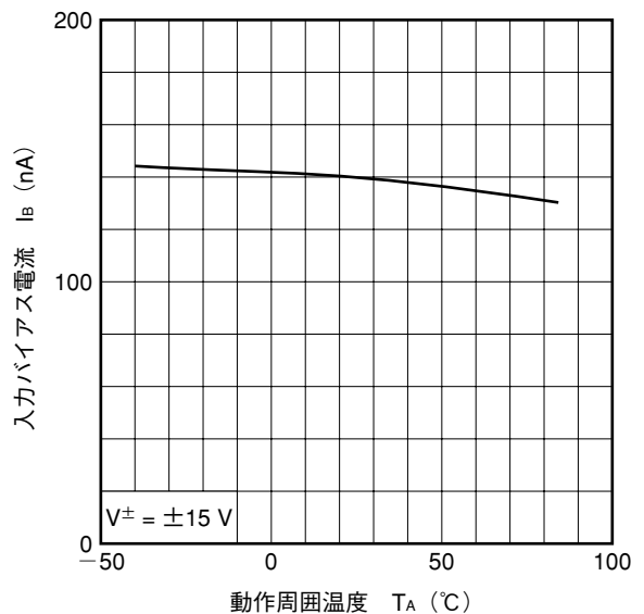
I B -T A 特性
