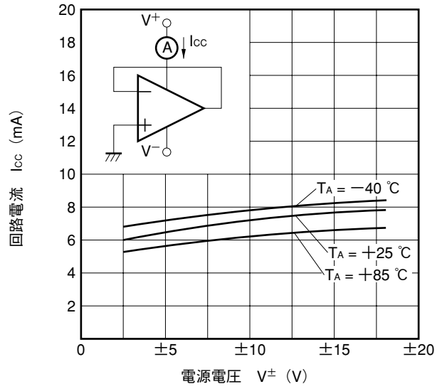
I CC -V ± 特性
