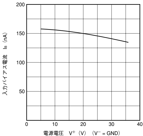
I B -V + 特性
