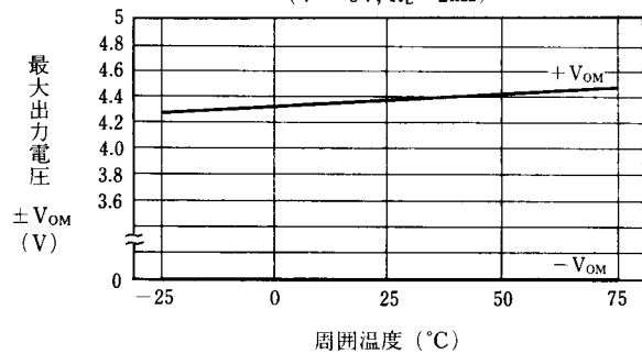
±最大出力電圧対周囲温度特性例 ( V^+ = 5V, R_L = 2k\Omega )
