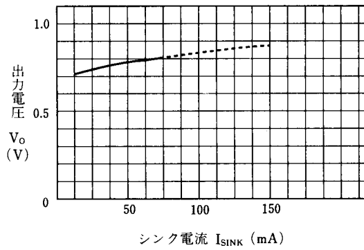
シンク電流特性例 ( V^+ = 5V , T_a = 25^\circ C )
