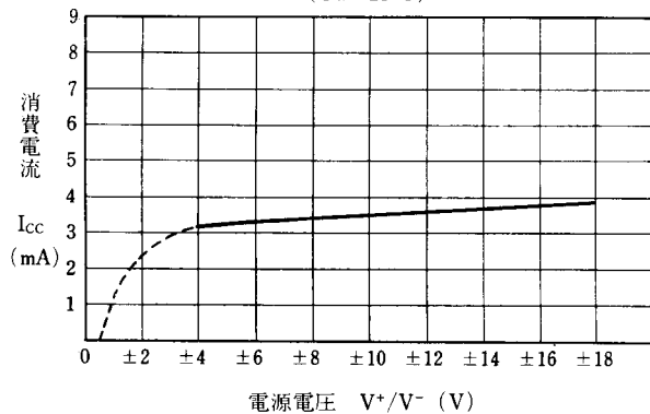
消費電流対電源電圧特性例 (Ta = 25°C)
