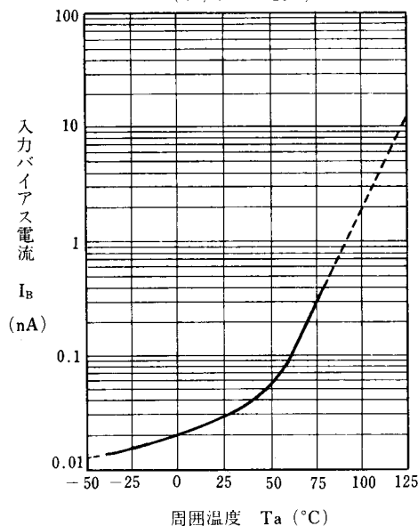
入力バイアス電流温度特性例 ( V^+/V^- = \pm 15V )
