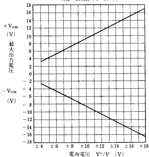
最大出力電圧対電源電圧特性例 (R L = 10kΩ, Ta = 25°C)
