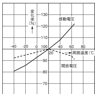
5. - (2) 周囲温度特性(1a1b, 2a)
