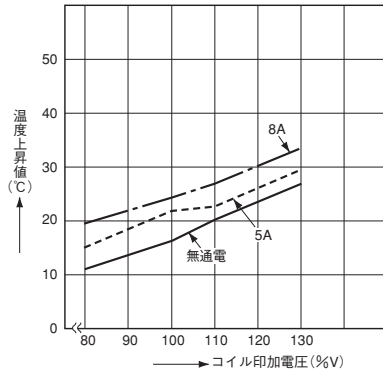
4. - (2) コイル温度上昇(1a1b, 2a)
