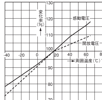
5. - (1) 周囲温度特性(1a)
