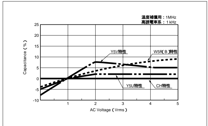
AC電圧特性
