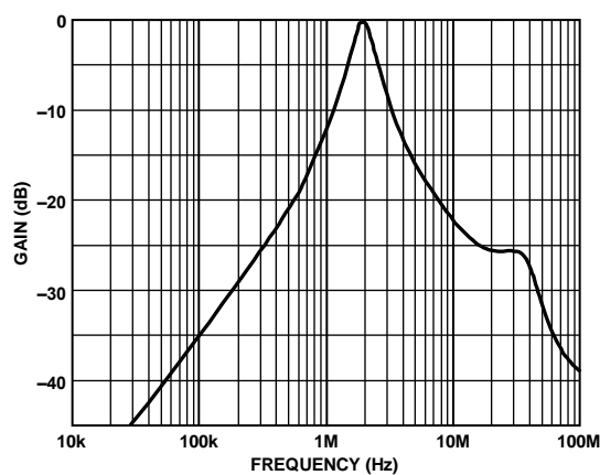
図 47. 2 MHz バンドパス・バイ・クワッド・フィルタの 周波数応答
