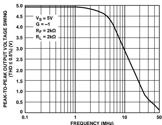
図 5. 低歪みのレール to レール出力振幅
