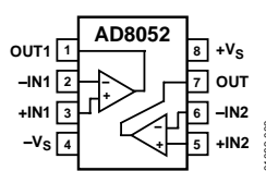
図 3. SOIC (R-8) と MSOP (RM-8)
