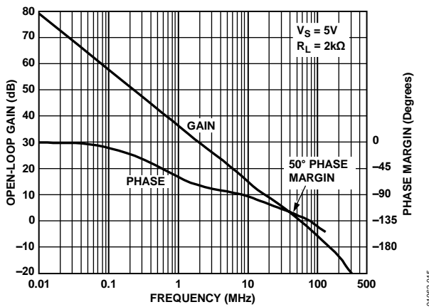
図 15. AD8051/AD8052 のオープン・ループ・ゲインと 位相の周波数特性
