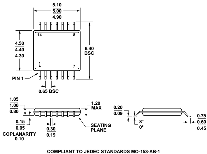
図 57.14 ピン薄型シュリンク・スモール・アウトライン・パッケージ[TSSOP] (RU-14) 寸法: mm
