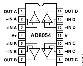
図 4. SOIC (R-14) と TSSOP (RU-14)
