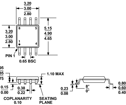
図 55.8 ピン・ミニ・スモール・アウトライン・パッケージ[MSOP] (RM-8) 寸法: mm
