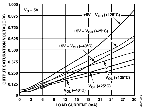
図 33. AD8054 の負荷電流対出力飽和電圧
