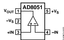
図 2. SOT-23-5 (RJ)
