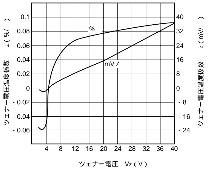
図4 Vz-z特性例
