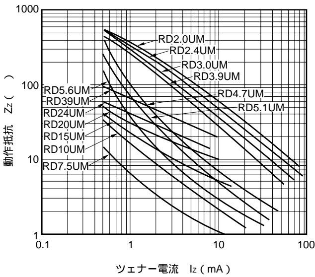
図3 Zz-iz特性例
