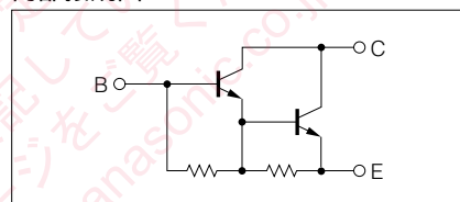
内部接続図
