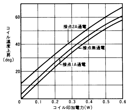
コイル温度上昇特性
