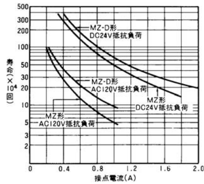
寿命曲線
