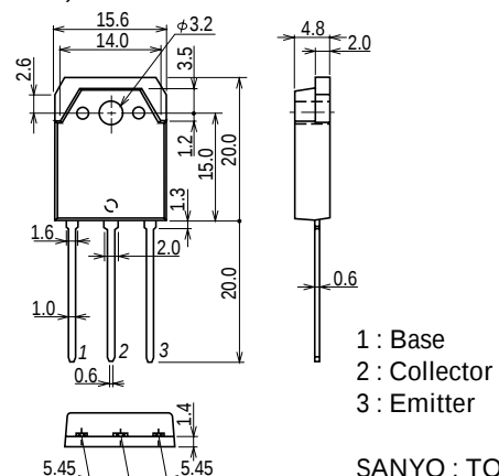
外形図 2022A (unit : mm)
