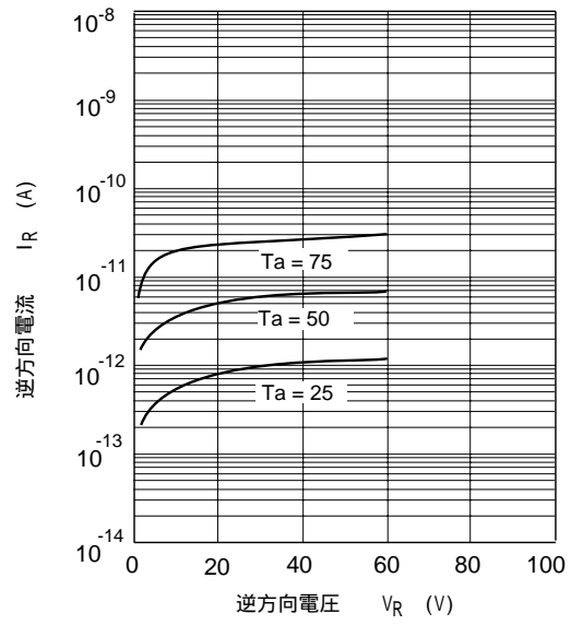
图2. 逆方向特性
