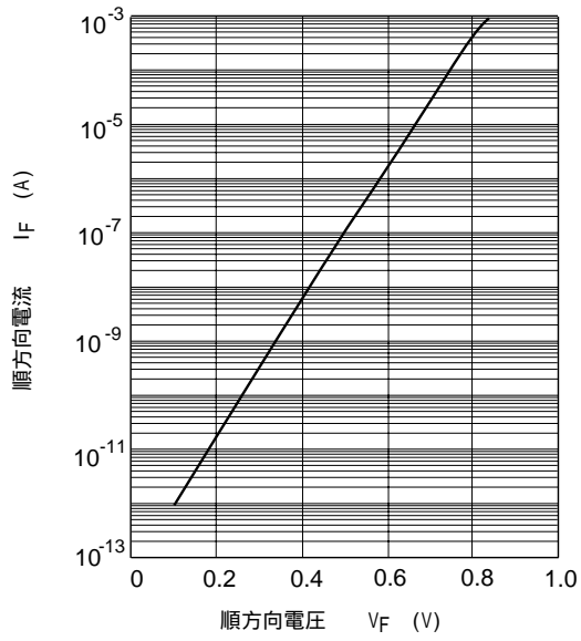
图1. 顺方向特性
