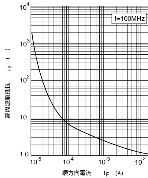
图4. 高周波顺抵抗 对 顺电流特性
