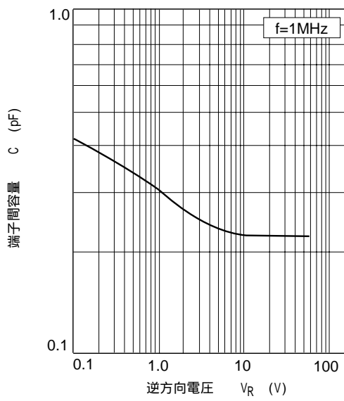
图3. 端子間容量 对 逆电压特性
