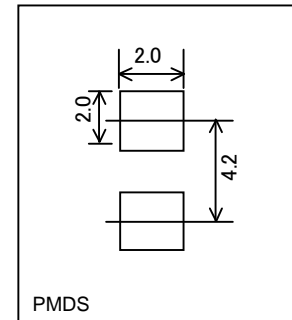
●ランド寸法図 (Unit : mm)
