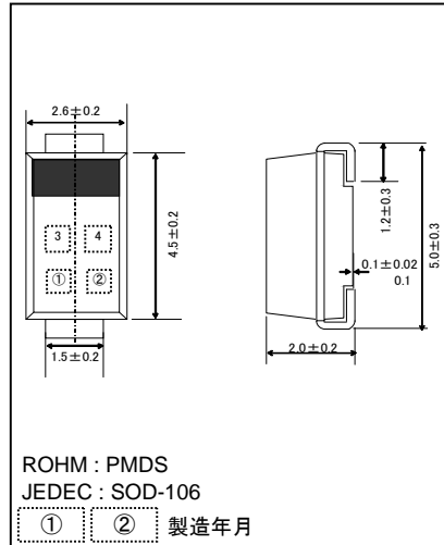
●外形寸法図 (Unit : mm)
