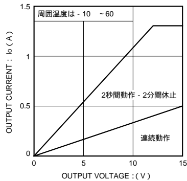
Fig.4 ディレーティングカーブ
