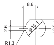
参考取付穴
