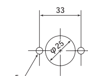
参考取付穴
