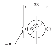
参考取付穴
