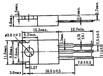
(JEDEC TO-220AB)
