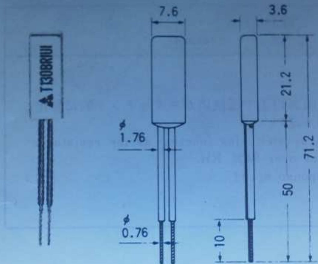
樹脂タイプ Resin Case Type
