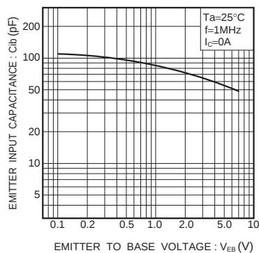
Fig.8 エミッタ入力容量 -エミッタ・ベース間電圧特性
