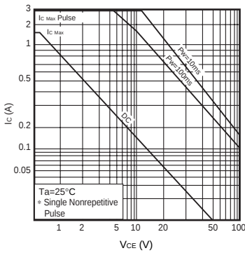
Fig.9 安全動作領域(2SD1867)
