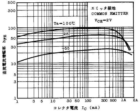
h_{FE} - I_C
