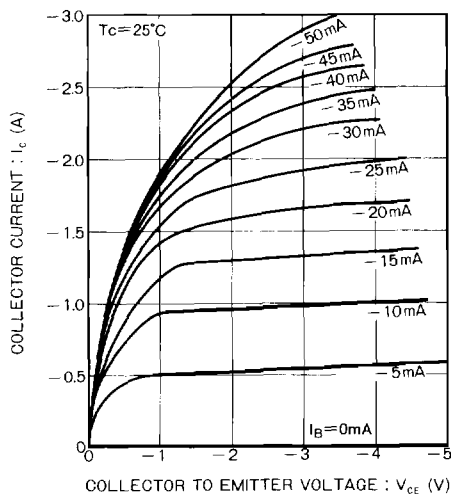
Fig. 5 エミッタ接地出力静特性
