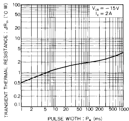
Fig. 3 過渡熱抵抗
